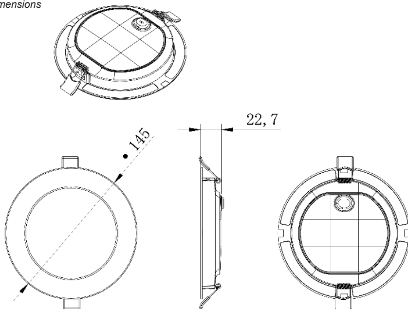
Dimensioni Dimensions
